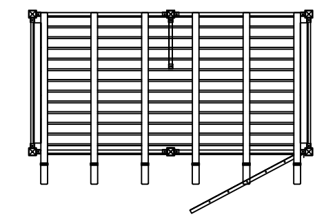
DTP-4 Top View SCALE: 3/8"=1'-0"
