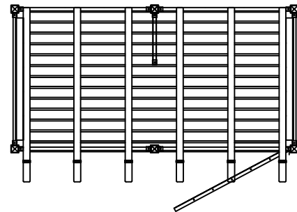
DTP-6 Top View SCALE: 3/8"=1'-0"
