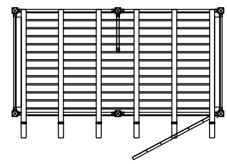
DTP-2 Top View SCALE: 3/8"=1'-0"
