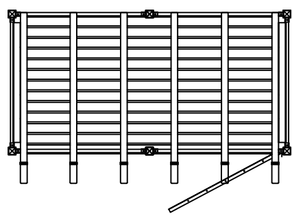
DTP-1 Top View SCALE: 3/8"=1'-0"
