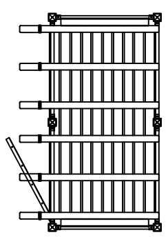
DTP-1 TOP VIEW N.T.S.
