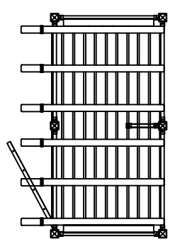
DTP-6 TOP VIEW N.T.S.
