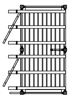
DTP-7 TOP VIEW N.T.S.
