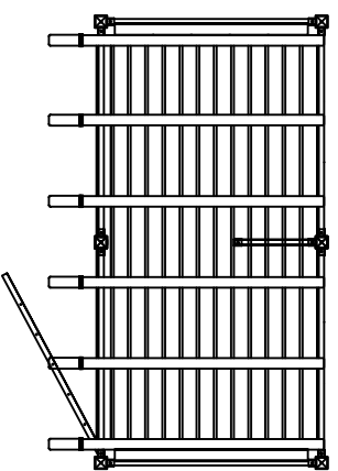
DTP-4 TOP VIEW N.T.S.
