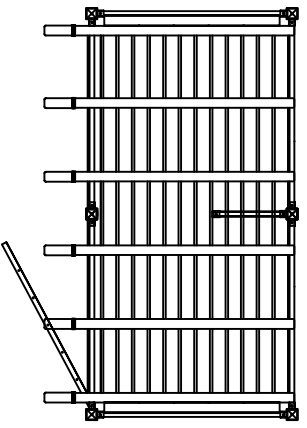
DTP-2 TOP VIEW N.T.S.
